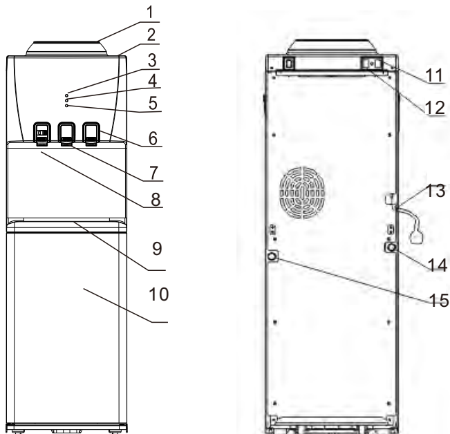
Мал. 1. Схема апарату CH-V130B
